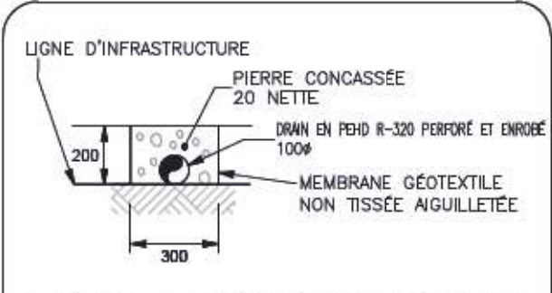
DÉTAIL - DRAIN DE FONDATION
